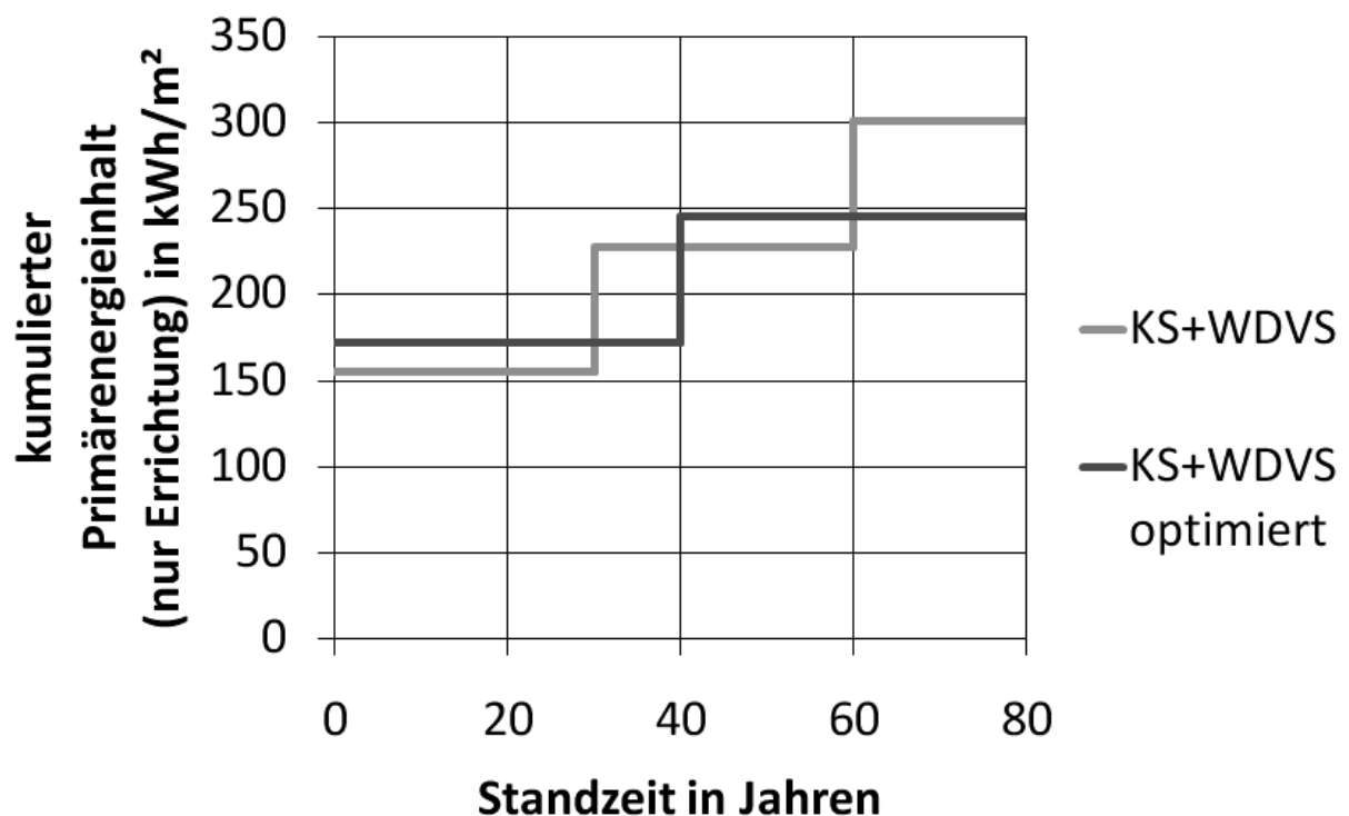
Bild 5: kumulierter Primärenergieeinhalt (hier nur Erstellungsphase)
