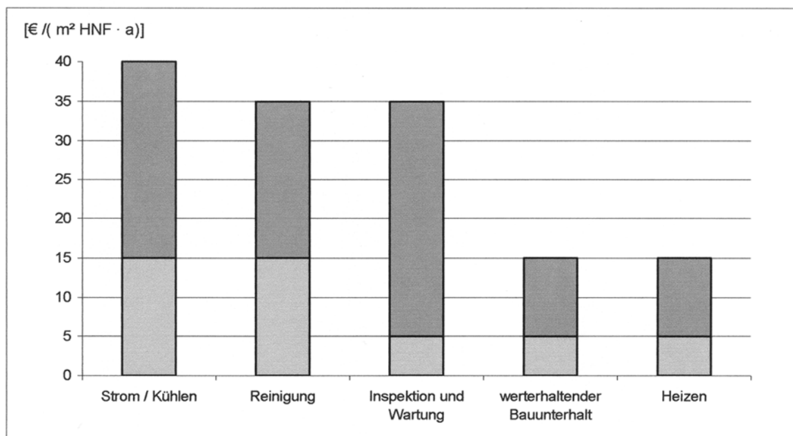
Bild 3: Betriebskosten (Ist-Werte) von Verwaltungsgebäuden
