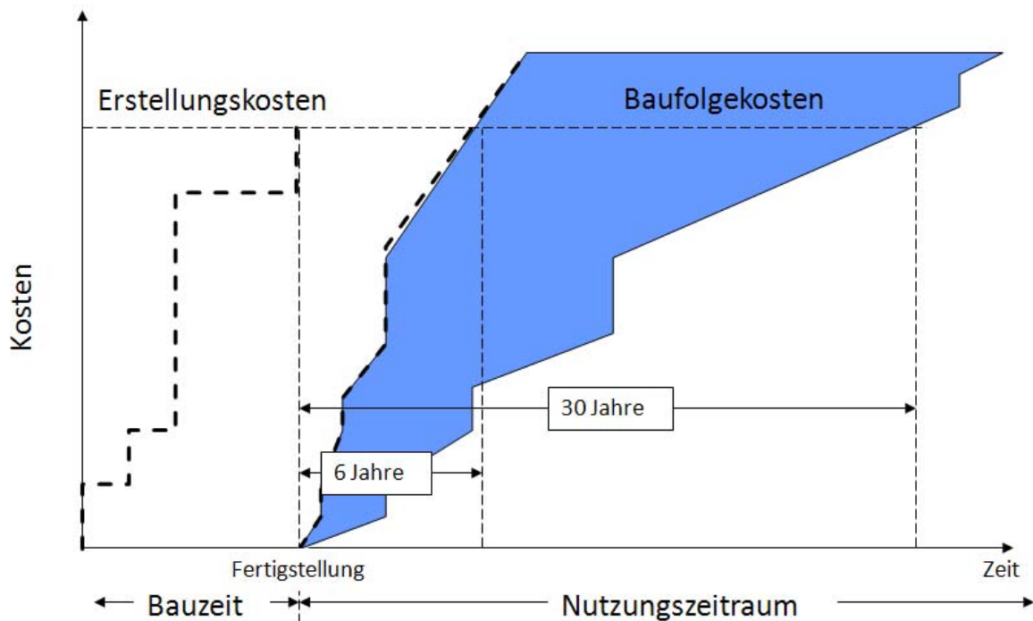
Bild 4: Errichtungs- und Betriebskosten [OFD Hannover]
