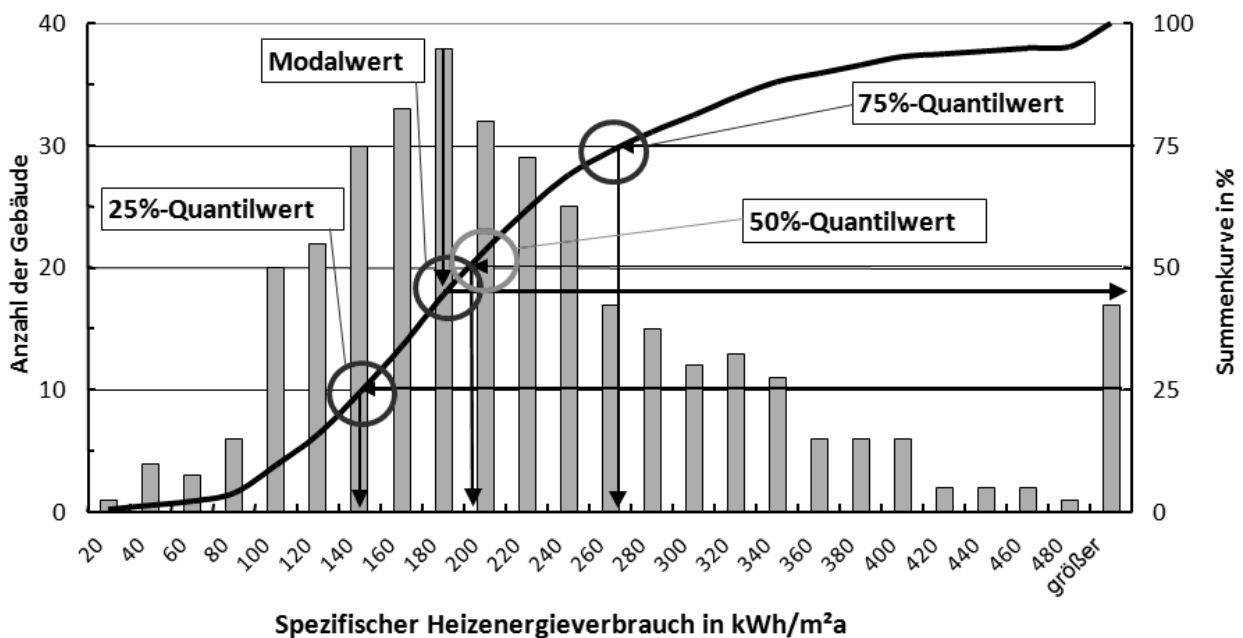
Bild 7: statistische Auswertung des spezifischen Heizenergieverbrauchs
